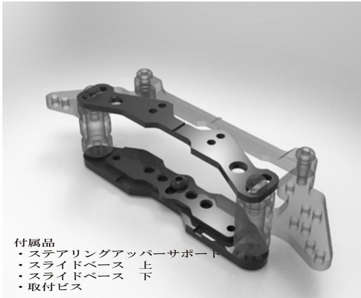
※2駆用クランク使用例
