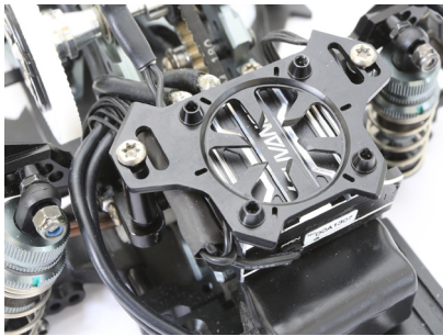
FAN無しでバックマウントV2使用に最適
